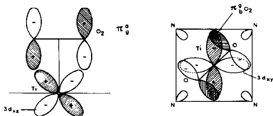
Fig. 7. Bonding scheme of the TiO_2 unit.
