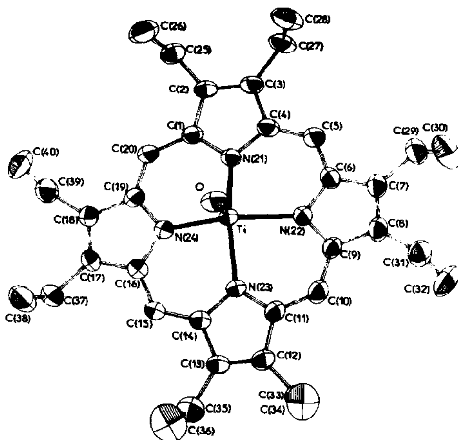
Fig. 3. ORTEP view of (OEP)Ti=O.
